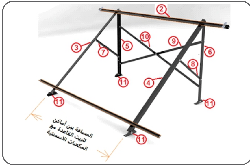
الشكل (٧): المسافة بين أماكن تثبيت القاعدة مع المكعبات الإسمنتية.
