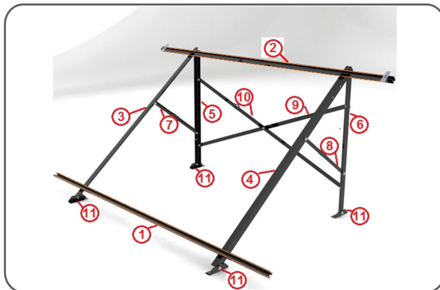
الشكل (١٢): أجزاء القاعدة المعدنية لأحد السخانات المستوردة.
