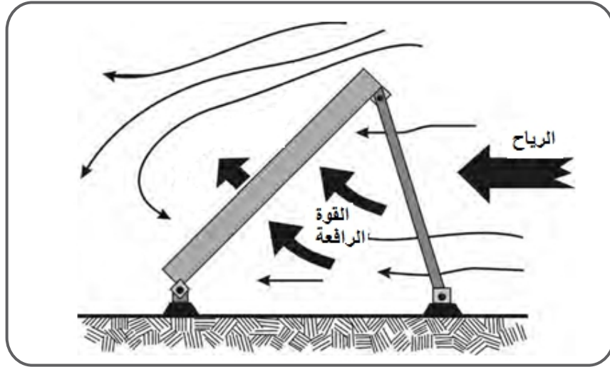
الشكل (٢): قاعدة السخان الشمسي.
